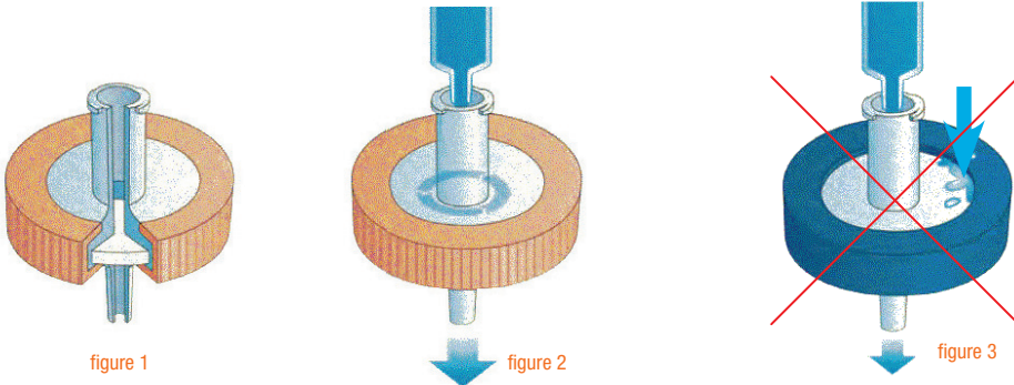
Figure 3. welded되지 않은 타사 Syringe Filter Leak 발생
